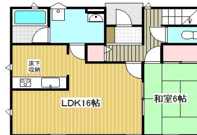
1階平面図
